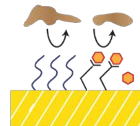
Antifouling membranes
