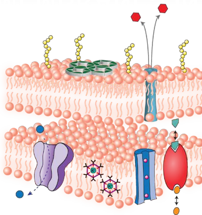
Cell membranes
